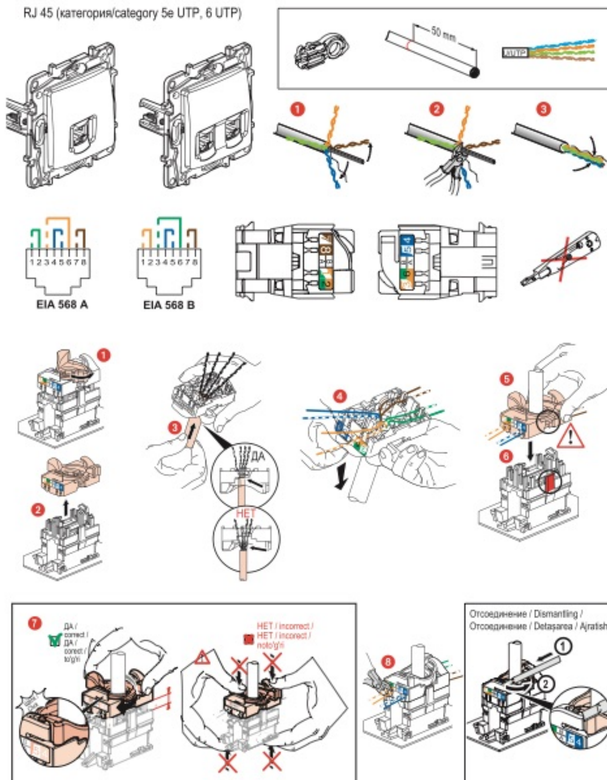
Рисунок 3 – Подключение компьютерных розеток RJ45 / Figure 3 – RJ45 computer socket-outlet connection / 3 сурет – RJ45 компьютерлік розеткаларды жалғай / Figura 3 – Conectarea prizelor pentru computer RJ45 / 3-rasm – RJ45 kompyuter rozetkalarini ulash
