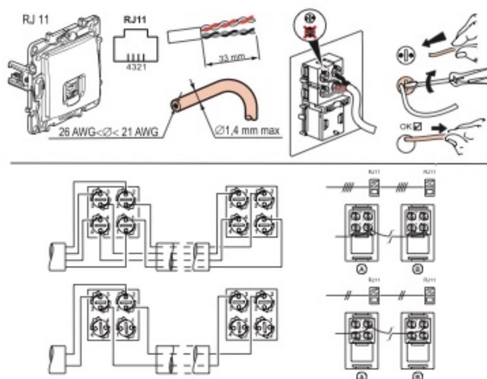
Рисунок 2 – Подключение телефонных розеток RJ11 / Figure 2 – RJ11 telephone socket-outlet connection / 2 сурет – RJ11 телефон розеткаларын жалғау / Figura 2 – Conectarea prizelor telefonice RJ11 / 2-rasm – RJ11 telefon rozetkalarini ulash
