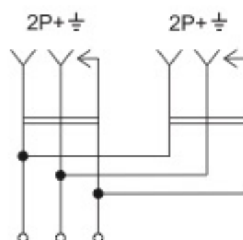
с) Розетка с заземлением двухместная Two-gang socket-outlet with ground contact / Жерге тұйықталған екі орынды розетка / Priză dublă cu împământare / Ikki o'rinli, yerga ulanishli rozetka
