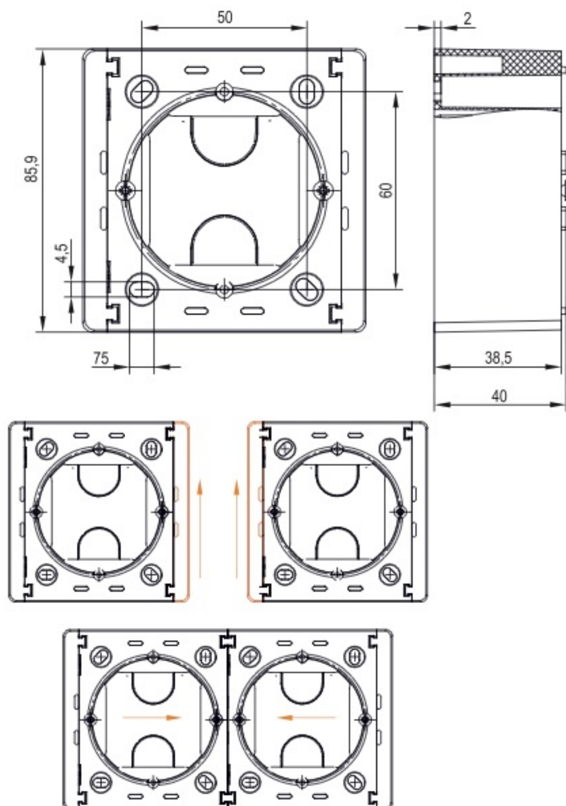
Рисунок 2 – Габаритные и монтажные размеры / Figure 2 – Overall and mounting dimensions / 2 сурет – Габариттік және монтаждау өлшемдері / Figura 2 – Dimensiuni totale și de instalare / 2-rasm – Gabarit va montaj o'lchamlari
