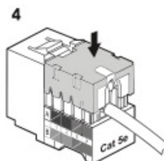
Рисунок 2 – Подключение компьютерной розетки RJ45 / Figure 2 – RJ45 computer socket-outlet connection / 2 сурет – RJ45 компьютерлік розеткаларды жалғау / Figura 2 – Conectarea prizelor pentru computer RJ45 / 2-rasm – RJ45 kompyuter rozetkalarini ulash
