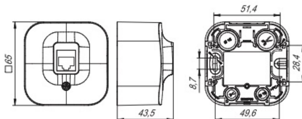
Рисунок 3 – Габаритные размеры / Figure 3 – Overall dimensions / 3 сурет – Габариттік өлшемдері / Figura 3 – Dimensiuni totale / 3-rasm – Gabarit o'lchamlari
