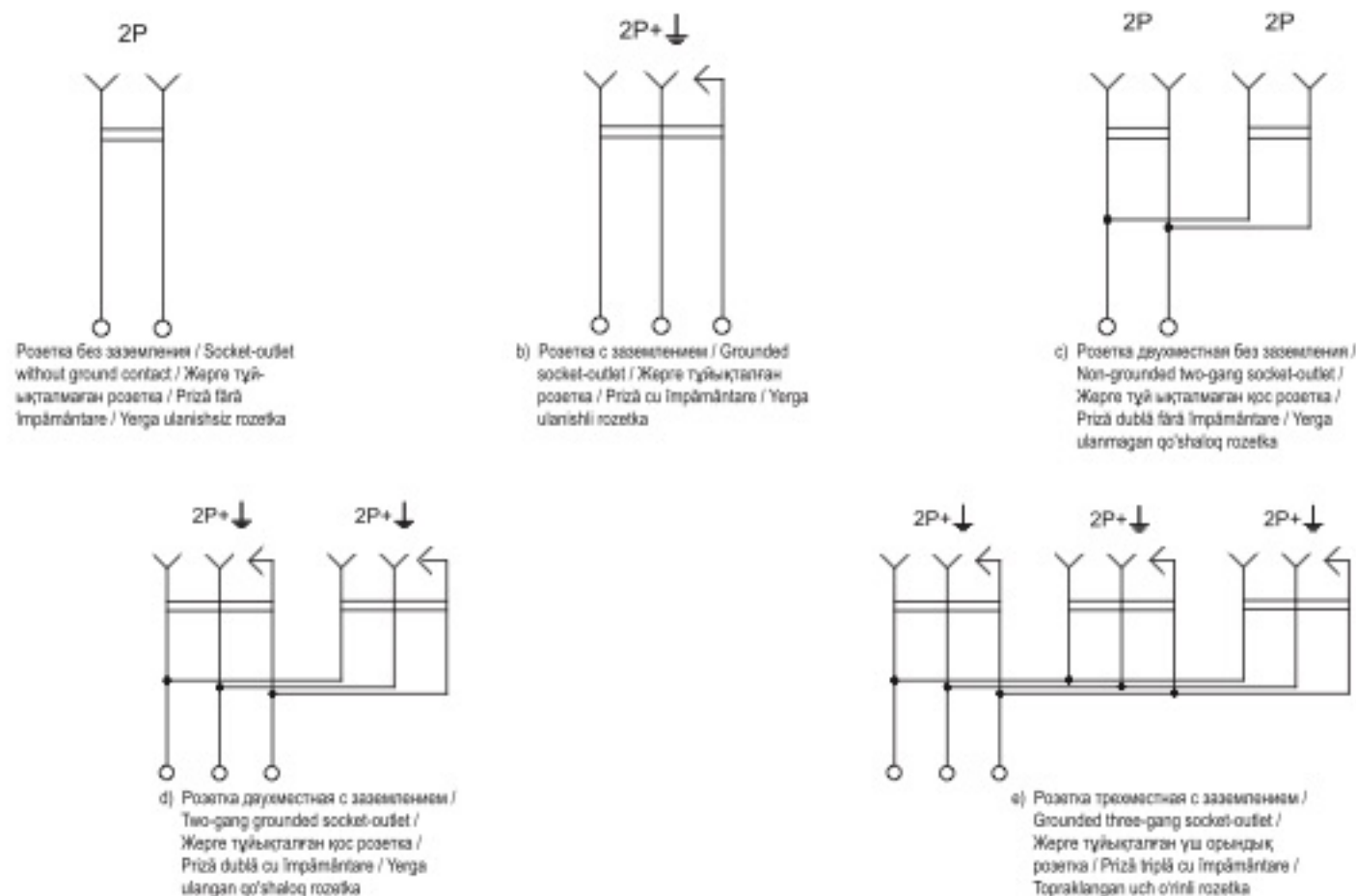
Рисунок 2 – Электрические схемы розеток / Figure 2 – Electrical diagrams of socket-outlets / 2 сурет – Розеткалардың электр схемалары / Figura 2 – Scheme electrice ale prizelor / 2-rasm – Rozetkalarining elektr sxemalari
