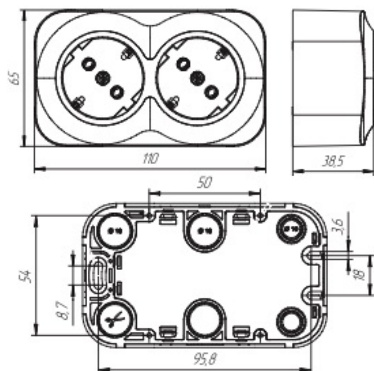
b) Розетка двухместная / Two-gang socket-outlet / Екі орындық розетка / Priză dublă / Qo'shaloq rozetka
