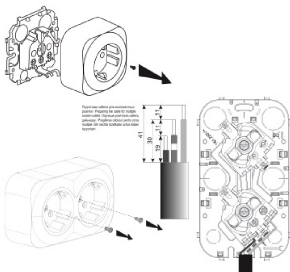
Рисунок 1 – Правила монтажа / Figure 1 – Installation rules / 1 сурет – Орнату ережелері / Figura 1 – Reguli de instalare / 1-rasm – O'rnatish qoidalari
