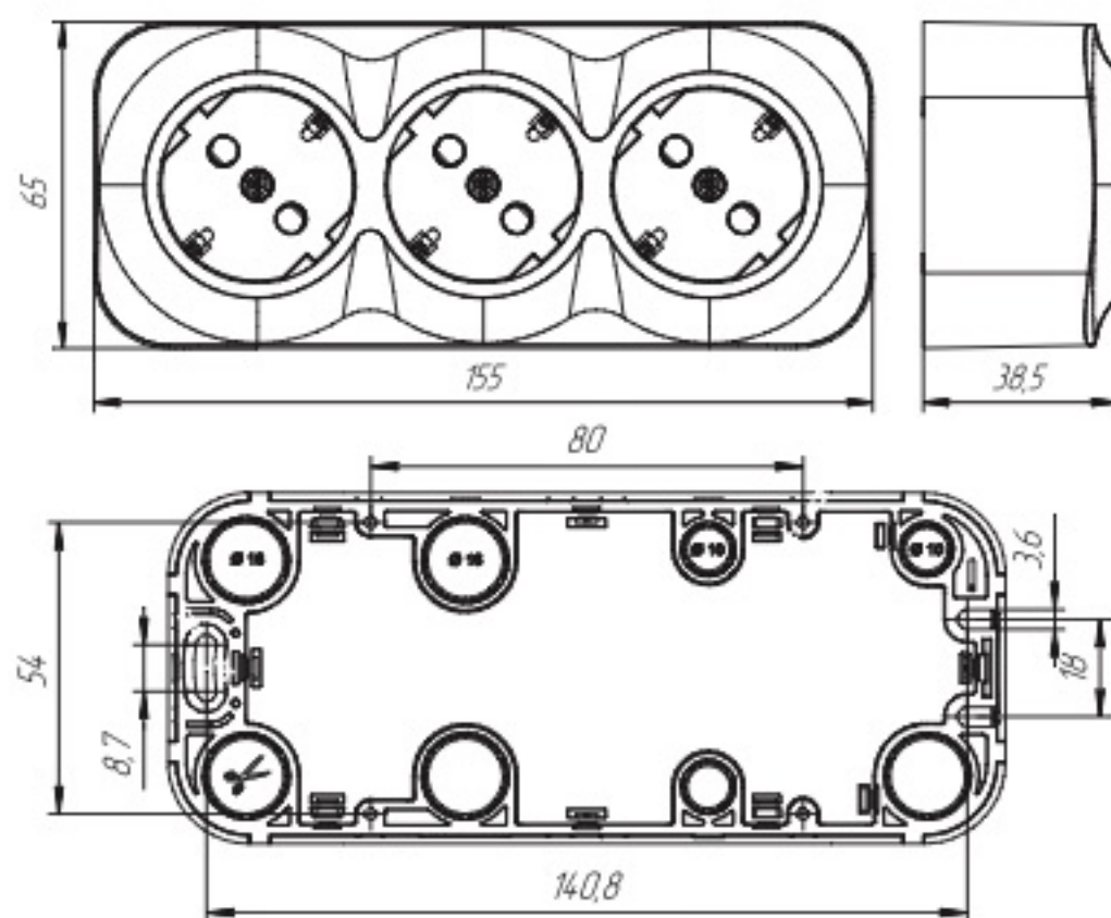
b) Розетка трехместная / Three-gang socket-outlet / Үш орындық розетка / Priză triplă / Uch o'rinni rozetka
