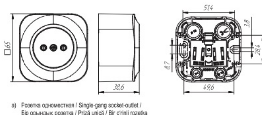
Рисунок 3 – Габаритные размеры розеток / Figure 3 — Overall dimensions socket-outlets / 3 сурет – Розеткаларының габариттік өлшемдері / Figura 3 – Dimensiuni totale ale prizelor / 3-rasm – Rozetkalarining gabarit o'lchamlari
