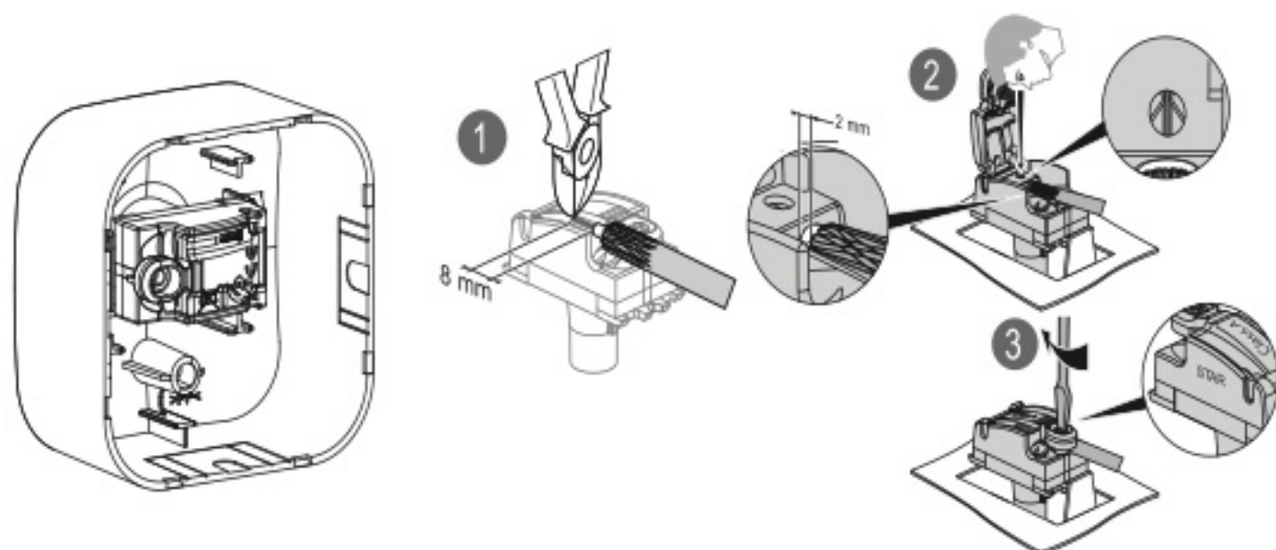
Рисунок 2 – Подключение телевизионной розетки / Figure 2 – TV socket-outlet connection / 2 сурет – Телевизиялық розетканы жалғай / Figura 2 – Conectarea prizei TV / 2-rasm – Televizion rozetkani ulash
