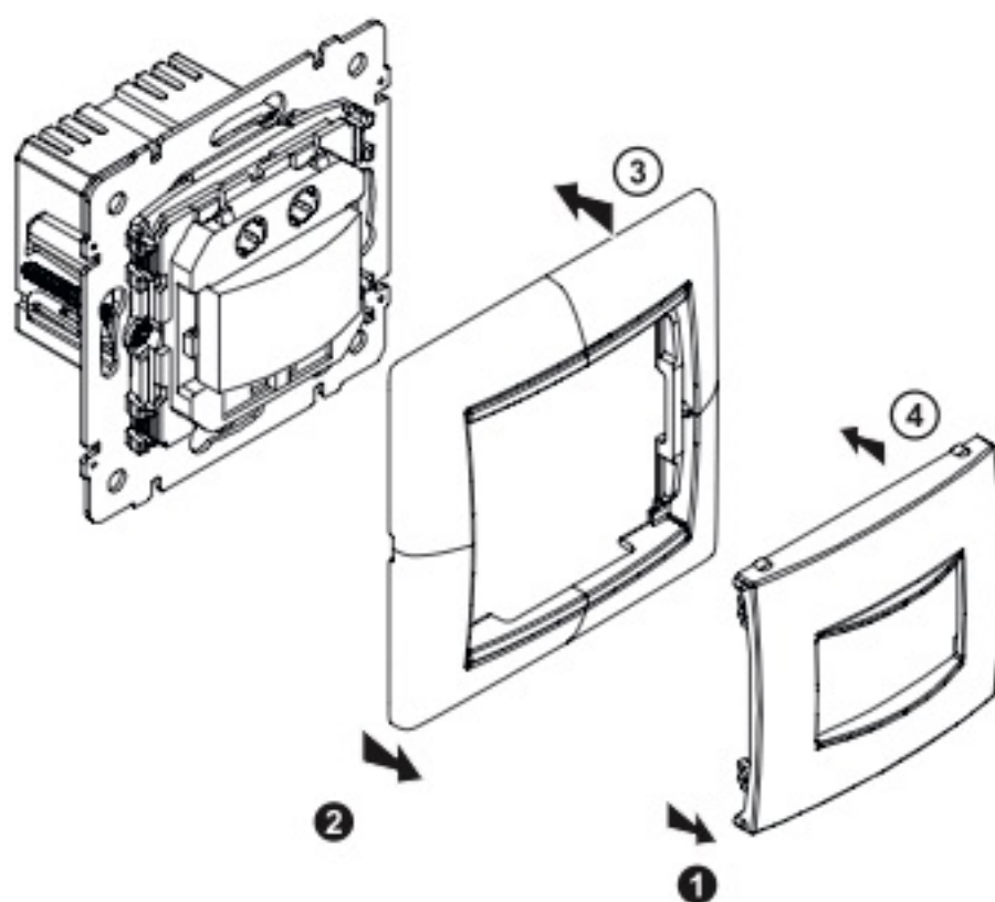
Рисунок 2 – Размещение датчика движения / Figure 2 – Placement of the motion sensor / 2 сурет – Қимыл датчигін орналастыру / Figura 2 – Amplasarea senzorului de mișcare / 2-rasm – Harakat datchigini joylashtirish
