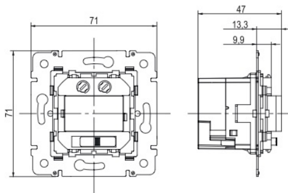
Рисунок 6 – Габаритные размеры / Figure 6 – Overall dimensions / 6 сурет – Габариттік өлшемдері / Figura 6 – Dimensiuni de gabarit / 6-rasm – Gabarit o'lchamlari
