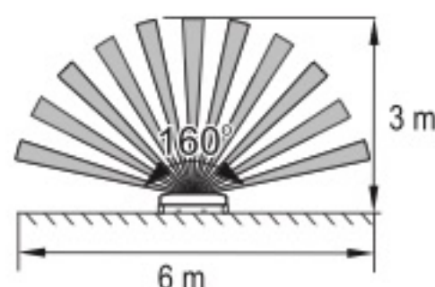
Размеры зоны / Detection range / Аймақтың өлшемдері / Dimensiunile zonei / Zona o'Ichami
