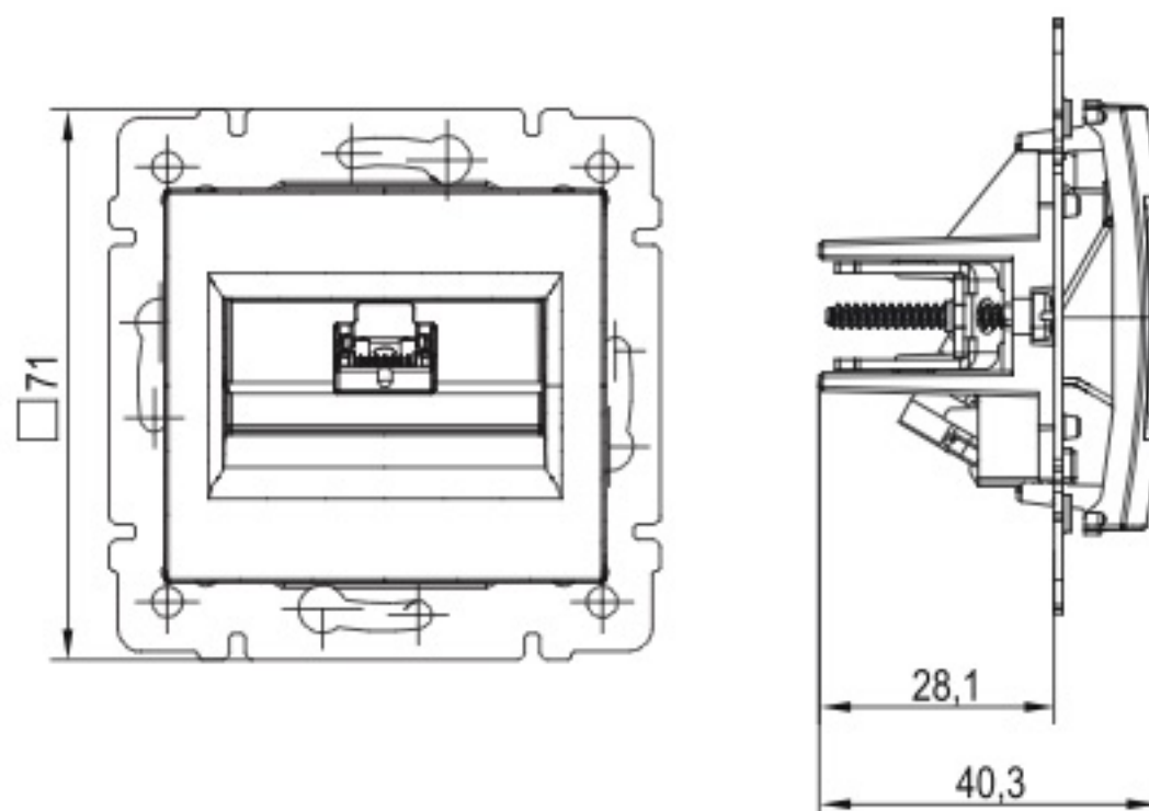
Рисунок 4 – Габаритные размеры телефонных розеток / Figure 4 – Overall dimensions of telephone sockets / 4 сурет – Телефон розеткалардың габариттік өлшемдері / Figura 4 – Dimensiunile generale ale prizelor telefonice / 4-rasm – Gabarit o'lchamlari
