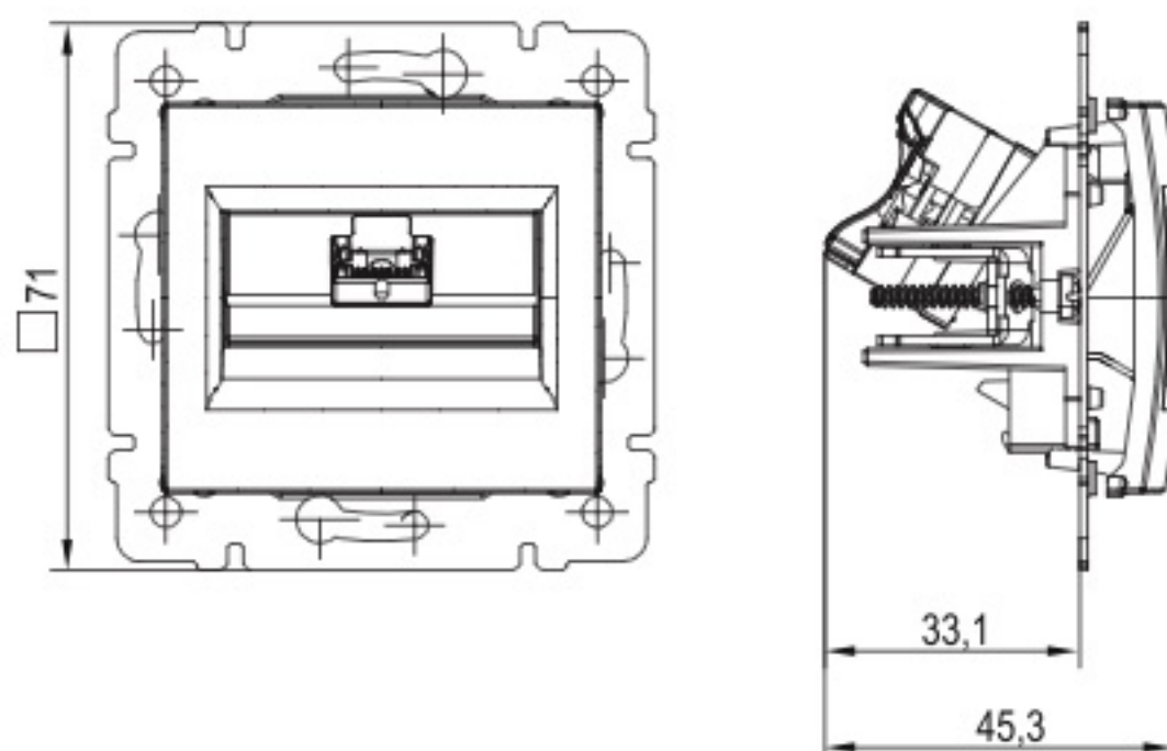
Рисунок 5 – Габаритные размеры компьютерных розеток / Figure 5 – Overall dimensions of computer sockets / 5 сурет – Компьютерлік розеткалардың габариттік өлшемдері / Figura 5 – Dimensiunile generale ale prizelor pentru computer / 5-rasm – Gabarit o'lchamlari
