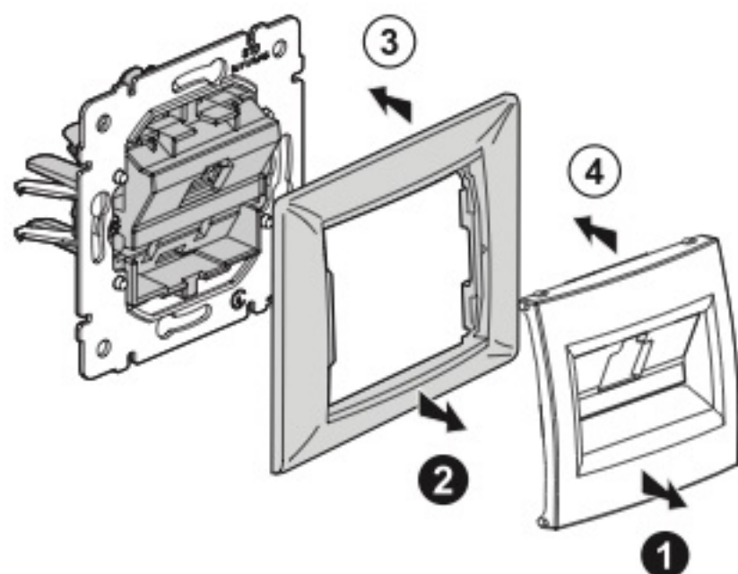
Рисунок 1 – Монтаж розетки / Figure 1 – Socket-outlet installation / 1 сурет – Розетканы монтаждау / Figura 1 – Instalarea prizei / 1-rasm – Rozetkani montaj qilish
